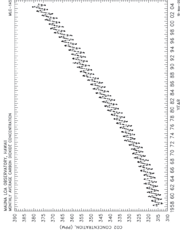
Figura 1 Crescita della concentrazione di CO 2 (ppm) in atmosfera - Osservatorio Mauna Loa, US
